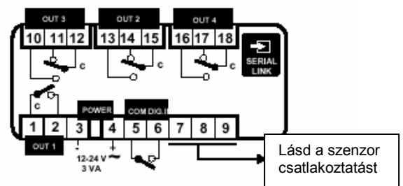
IR32Z – Pt100, J/K vagy V/I bemenettel
